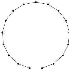
1. ábra. Szabályos 17-szög
